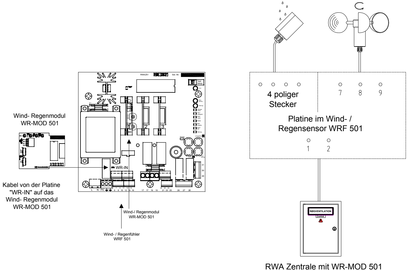
Abbildung 10: Anschluss Wind-/ Regenauswertung WRA 501
