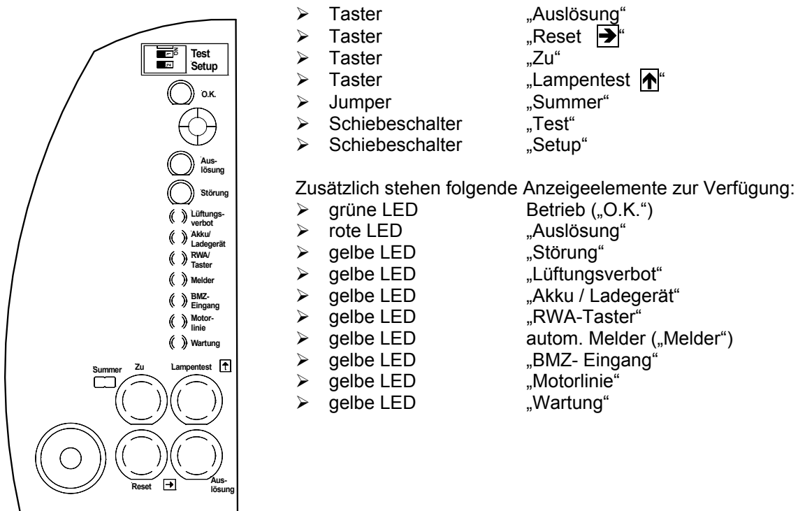
Abbildung 16: Anzeige- und Bedienelemente
